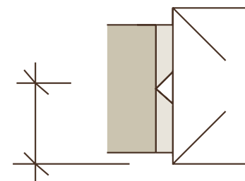
ca. 80 mm zwischen Außenkante Balken und Mitte Dreiecksleiste
