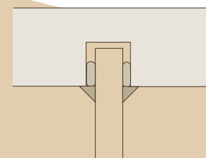
Dichten mit Stopfwolle und Lehmklebe- und Armierungsmörtel (auf dem Holz ggf. mit Putzträger)
