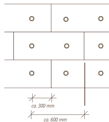
Schraubenabstand, Plattenabstand
