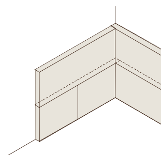
Verzahntes Versetzen in Raumecken
