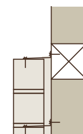
Befestigung der Vormauerschale
