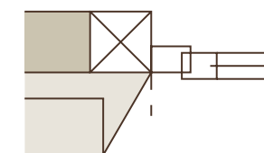
Fensteranschluss \leq 30^\circ
